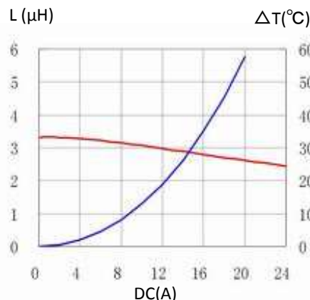
9. 125CDMCCDS-3R3MC
