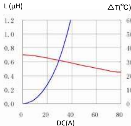
3. 125CDMCCDS-R68MC
