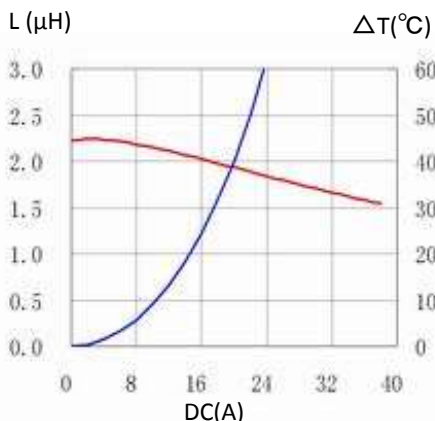
8. 125CDMCCDS-2R2MC
